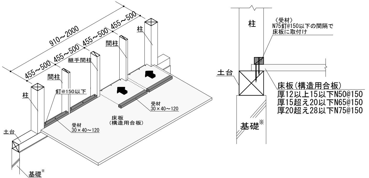
垂直断面図
