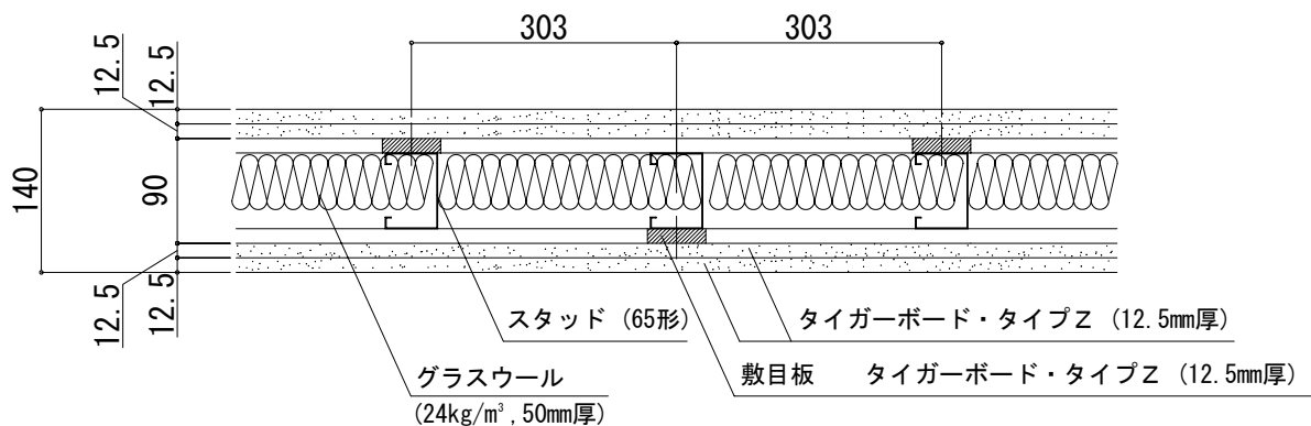
水平断面図 (TL D -50の遮音性能とする場合の壁構造)
