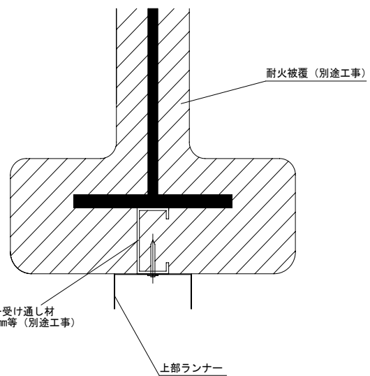
<鉄骨梁へのランナーの取り付け>
