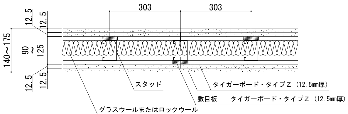
水平断面図 (認定の仕様)
