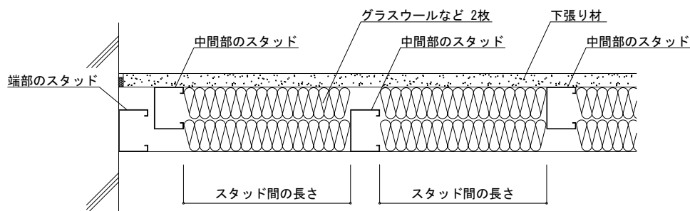
<グラスウールなどの挿入例>
