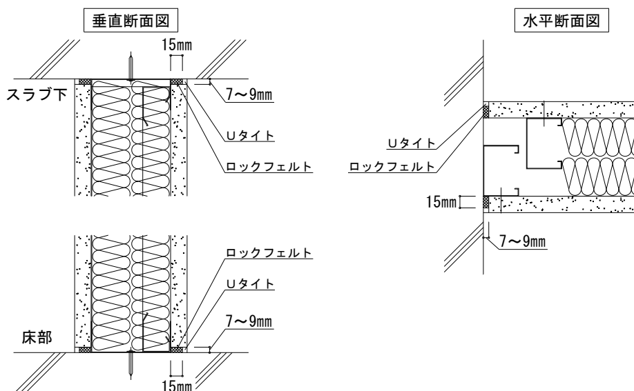
<スラブ下および床部の納まり例>
