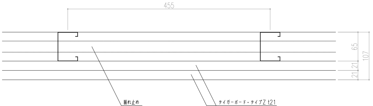
壁高さと同製下地材の選定例
