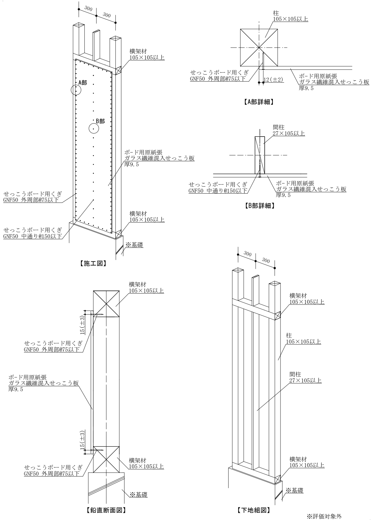
図4 施工詳細図 (寸法単位: mm)
