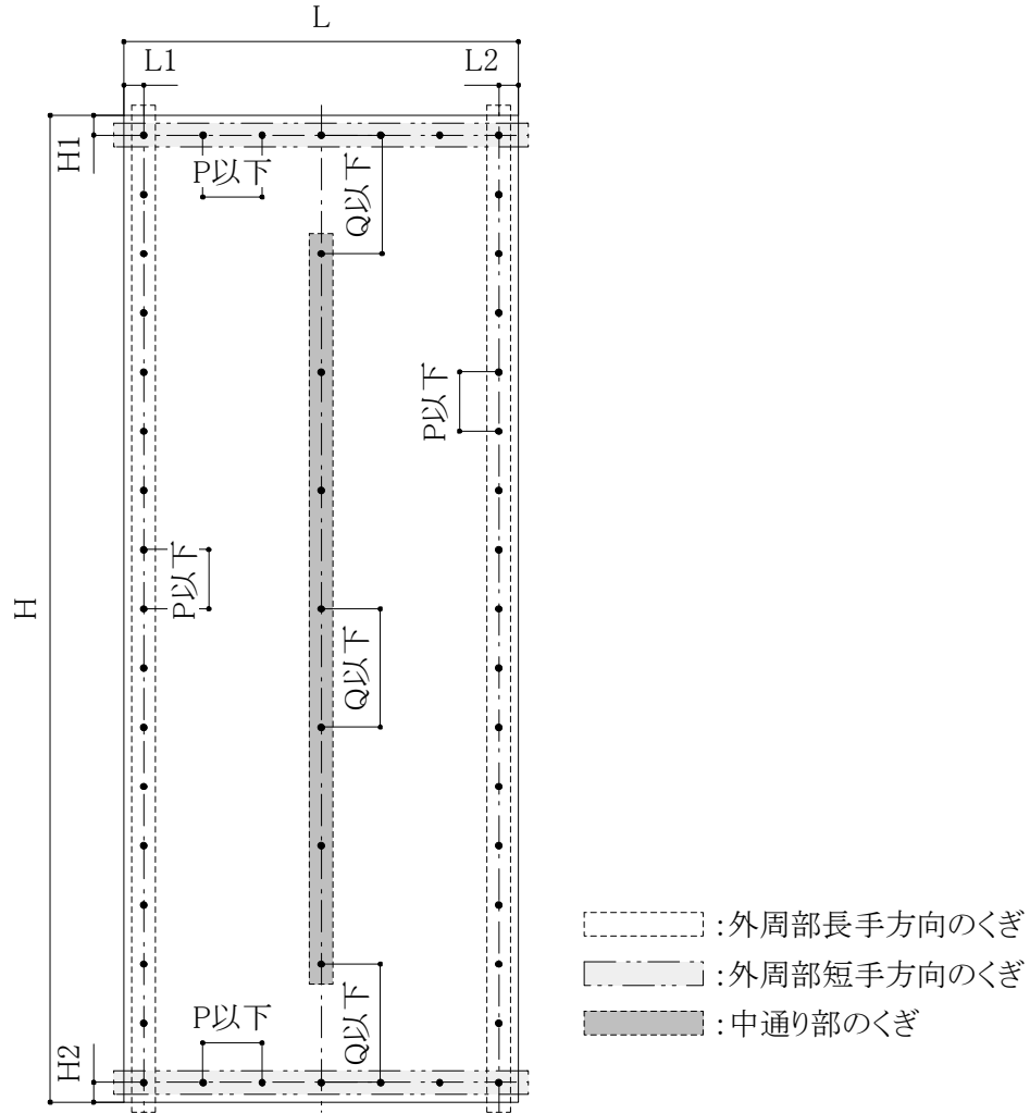
図3 各部のくぎ本数
