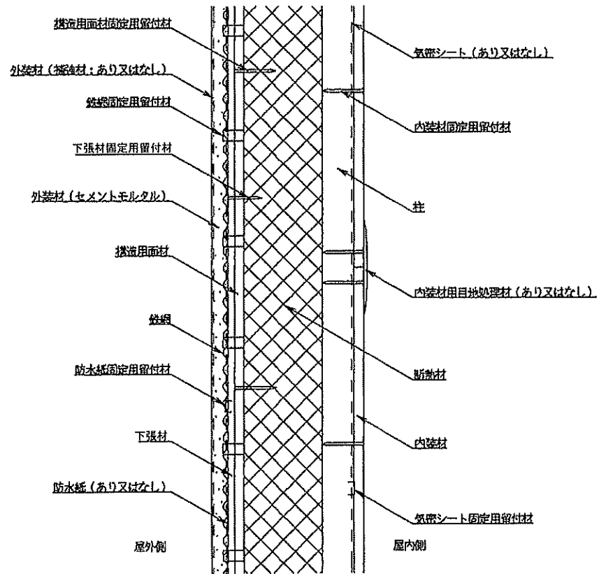
鉛直断面
