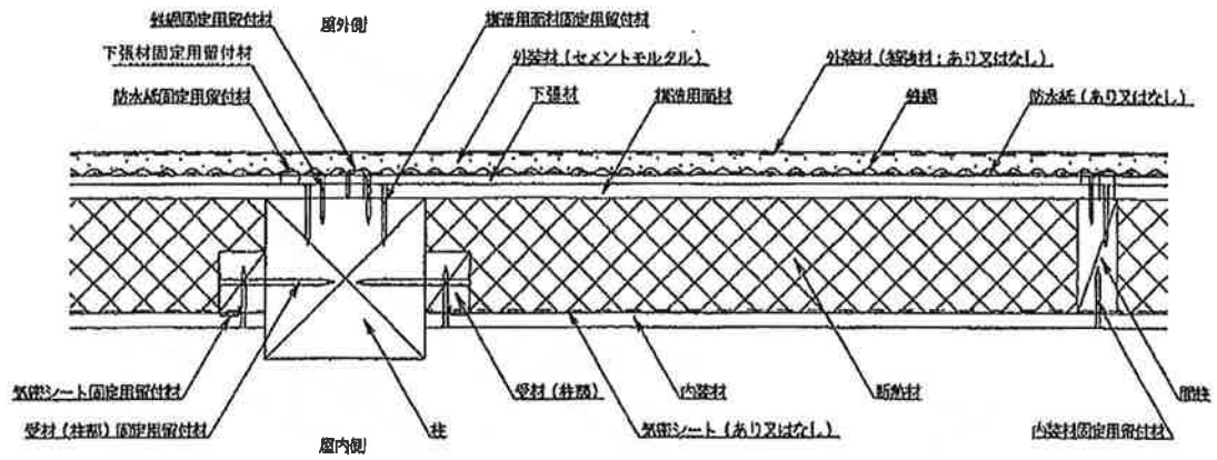
水平断面
