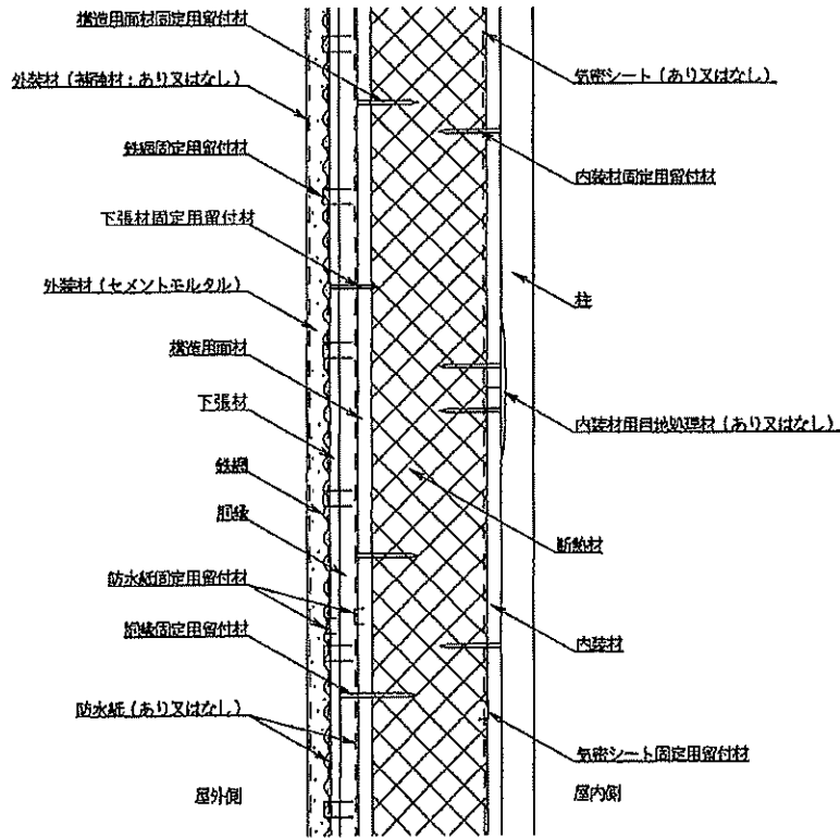
鉛直断面
