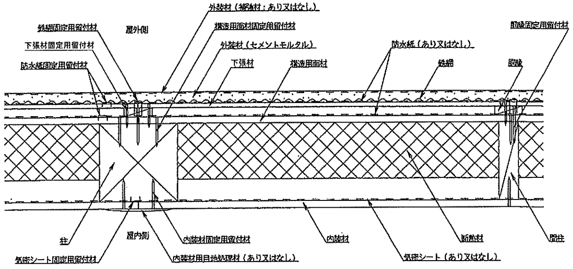
水平断面
