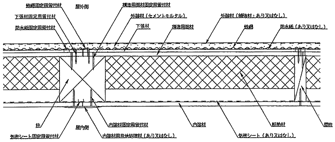
水平断面
