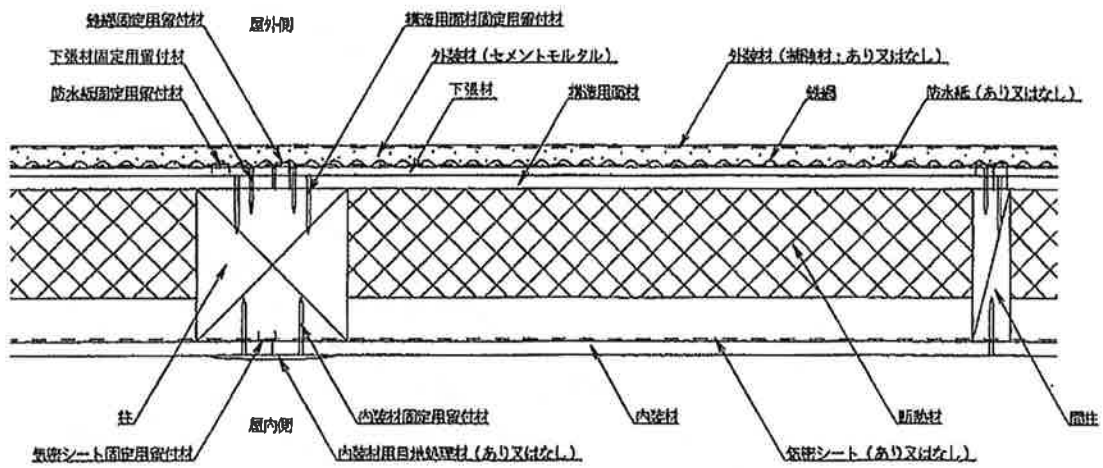
水平断面
