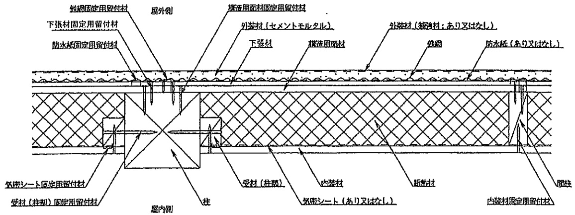
水平断面
