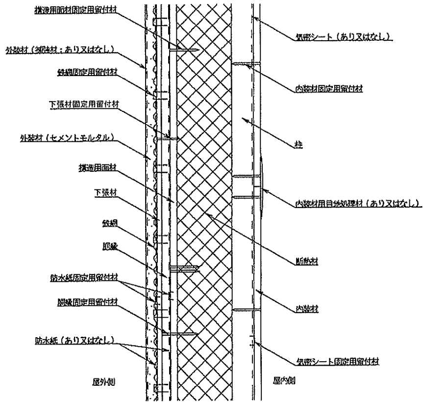
鉛直断面
