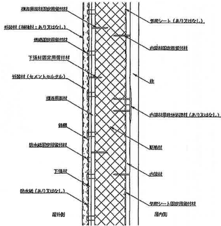
鉛直断面
