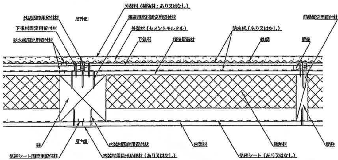
水平断面
