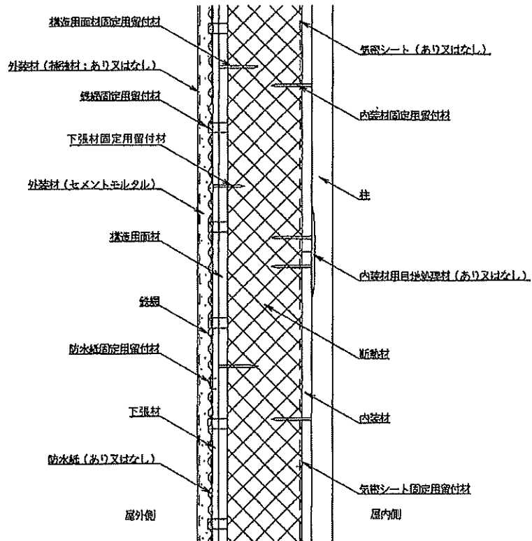
鉛直断面
