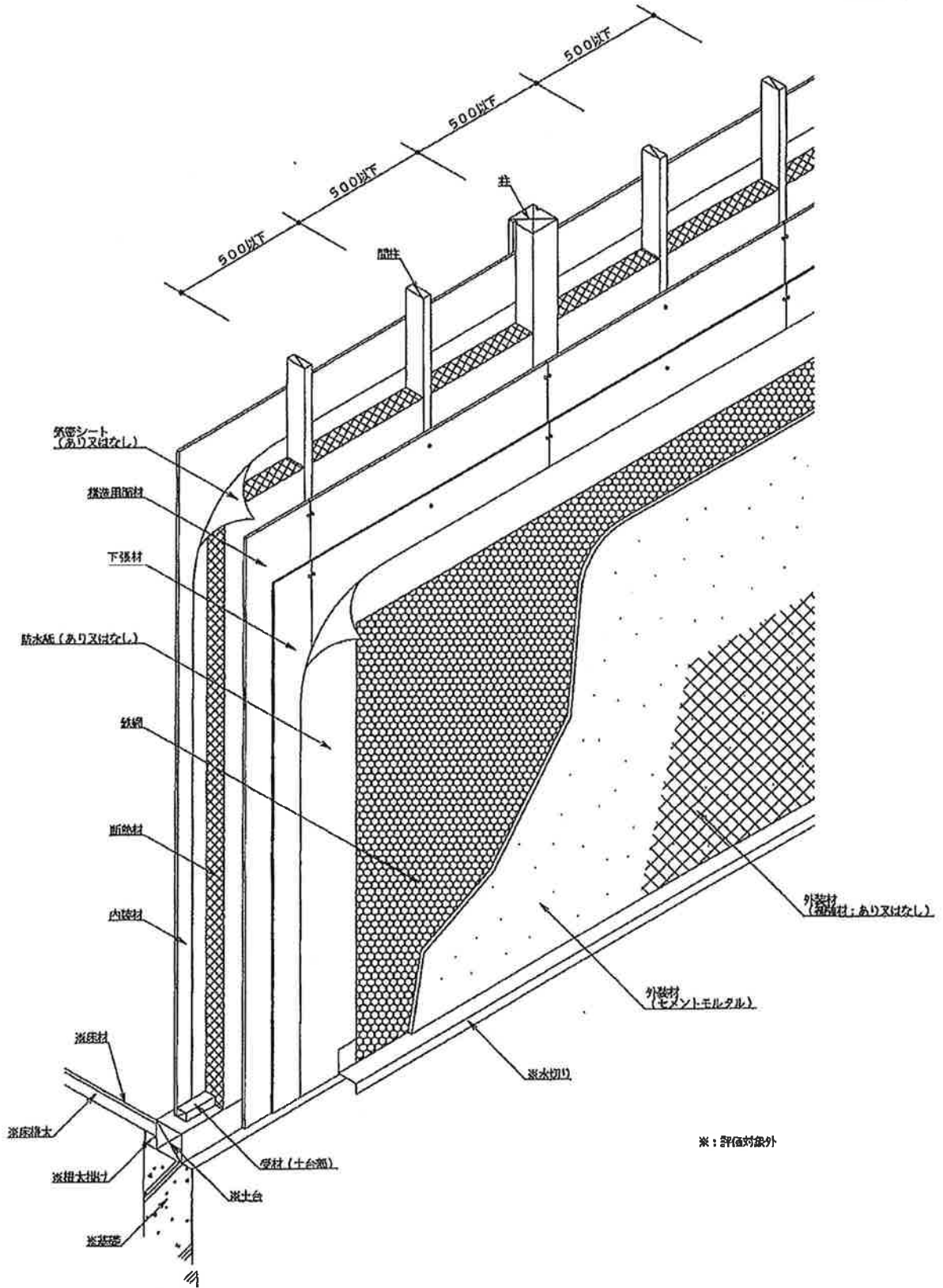
図1 構造説明図 透視図(欠き込み真壁造:直張仕様) (構造用面材あり/下張材あり)
