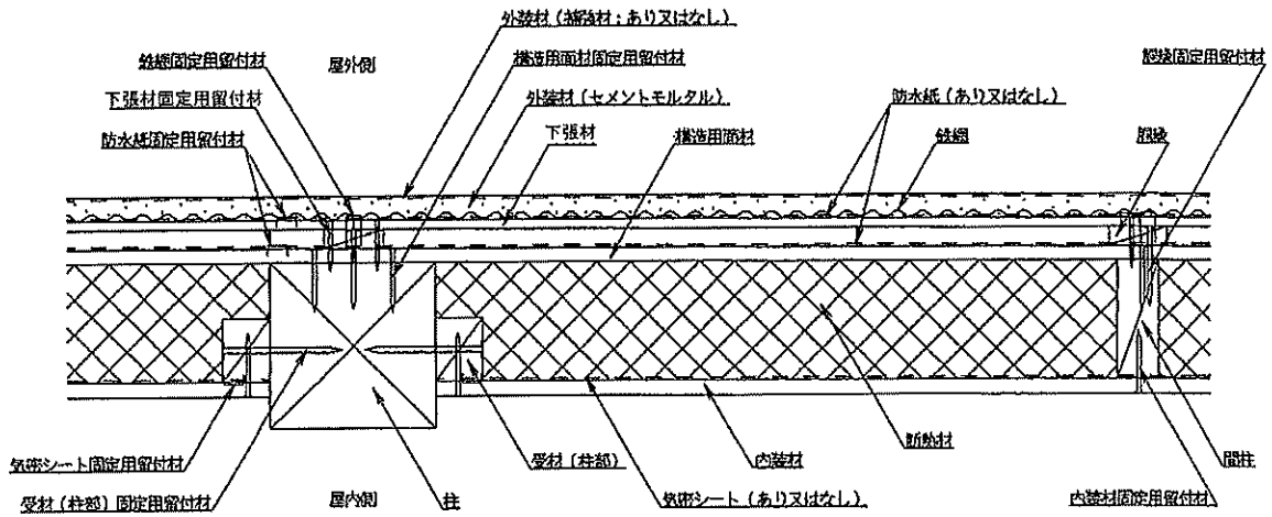
水平断面
