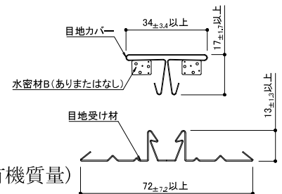
目地カバーと目地受け材の代表例
