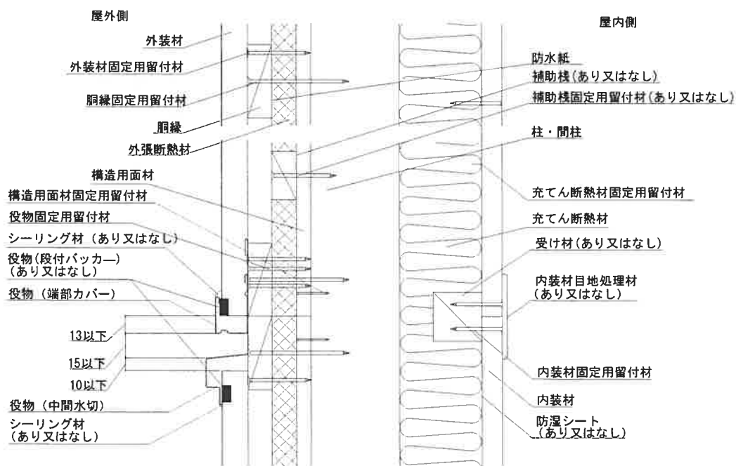
鉛直断面図
