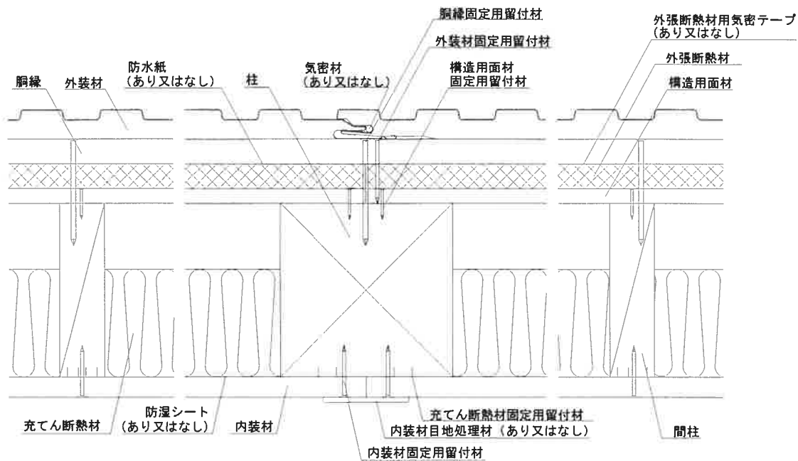
水平断面図
