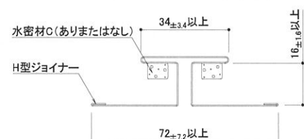
H型ジョイナーの代表例
