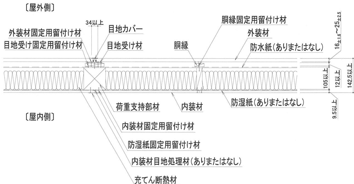
水平断面図(横張(構造用面材なし)の場合)
