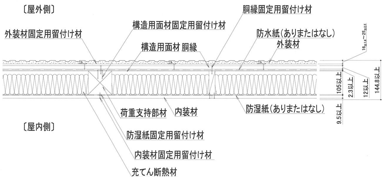
水平断面図(縦張(構造用面材あり)の場合)
