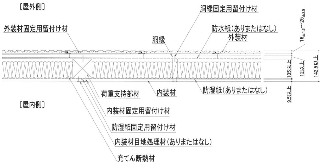
水平断面図(縦張(構造用面材なし)の場合)
