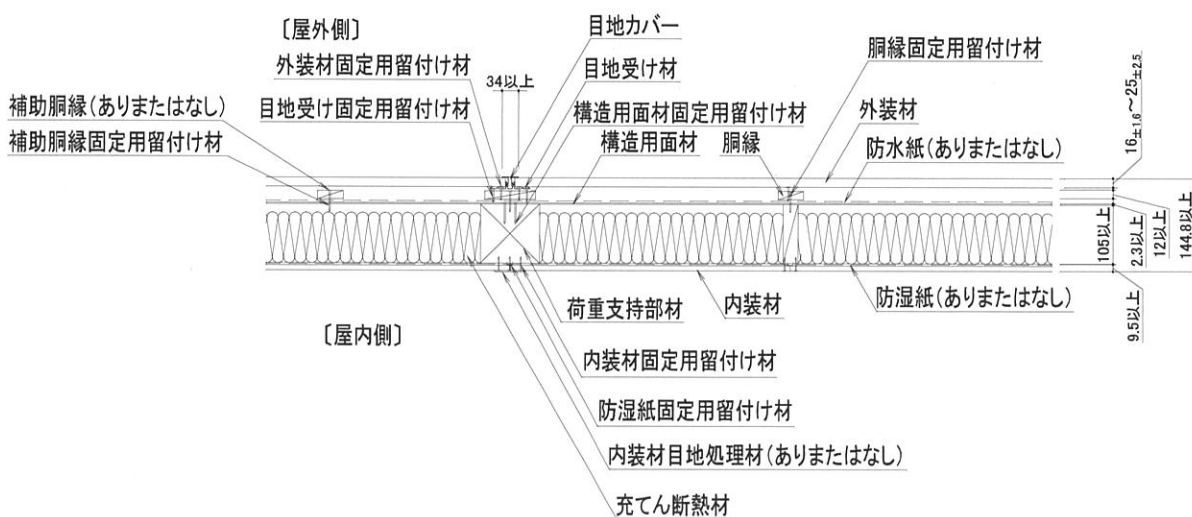
水平断面図(横張(構造用面材あり)の場合)
