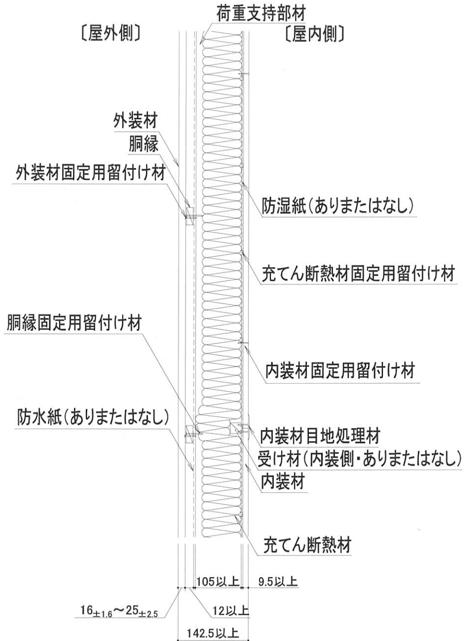
鉛直断面図(縦張(構造用面材なし)の場合)
