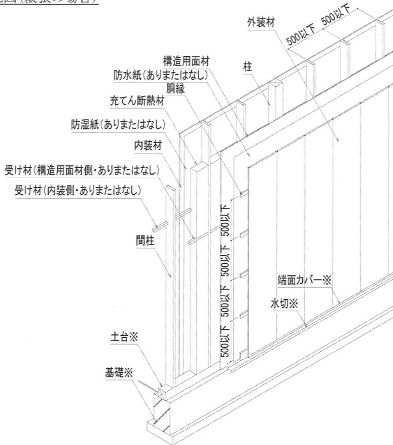
斜視図(縦張の場合)
