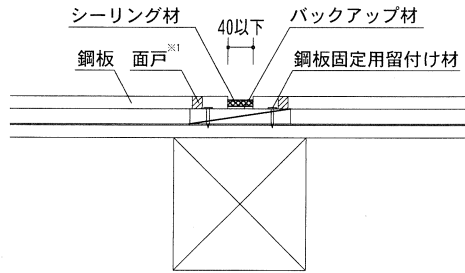
④ 目透かし目地
