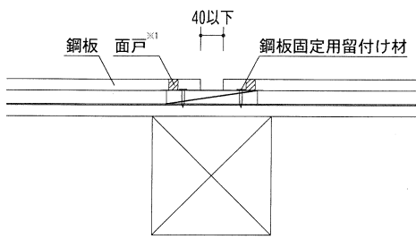
③ 目透かし目地
