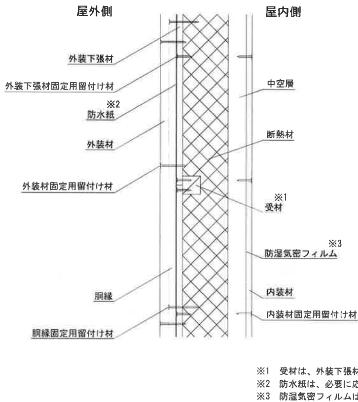
図-4 断面図 (外装材縦張仕様 (銅縁 縦張))
