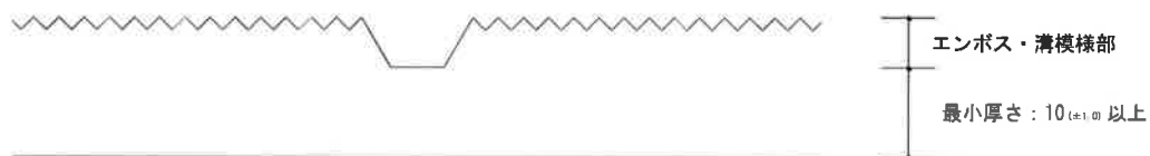
図- 8 外装材の端部形状及び断面形状の概略図
