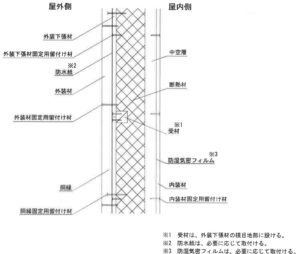
図-4 断面図 (外装材縦張仕様 (胴縁 縦張))
