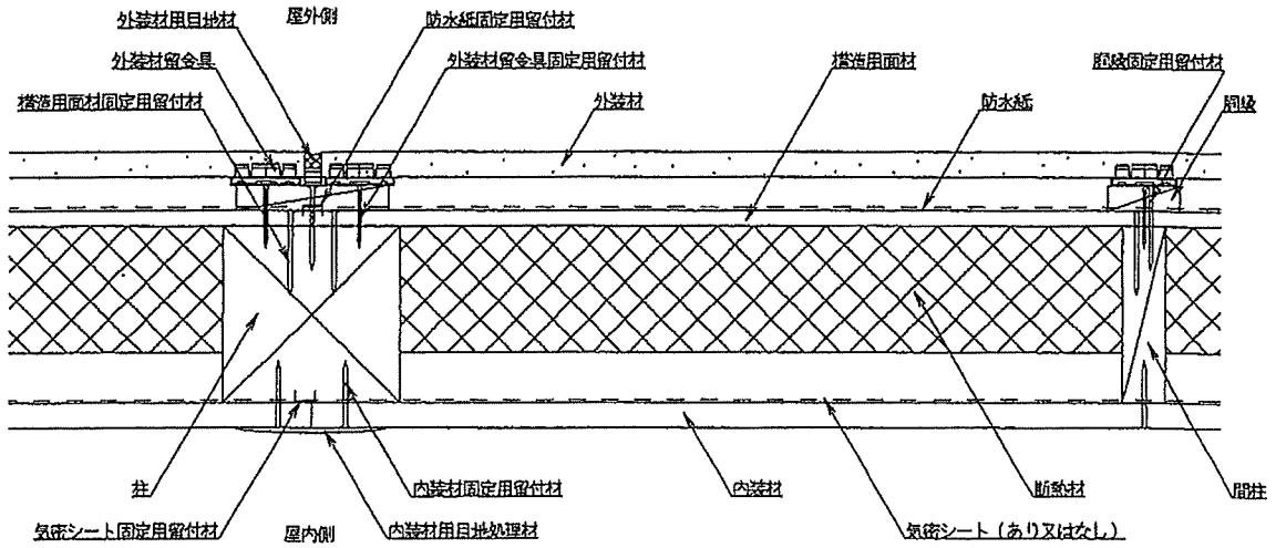
水平断面図
