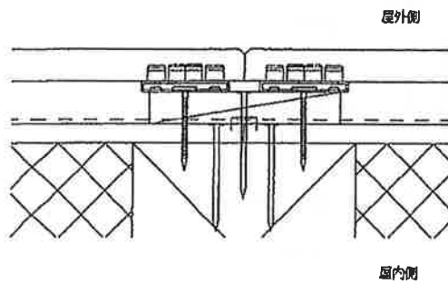
⑤突き付け目地
