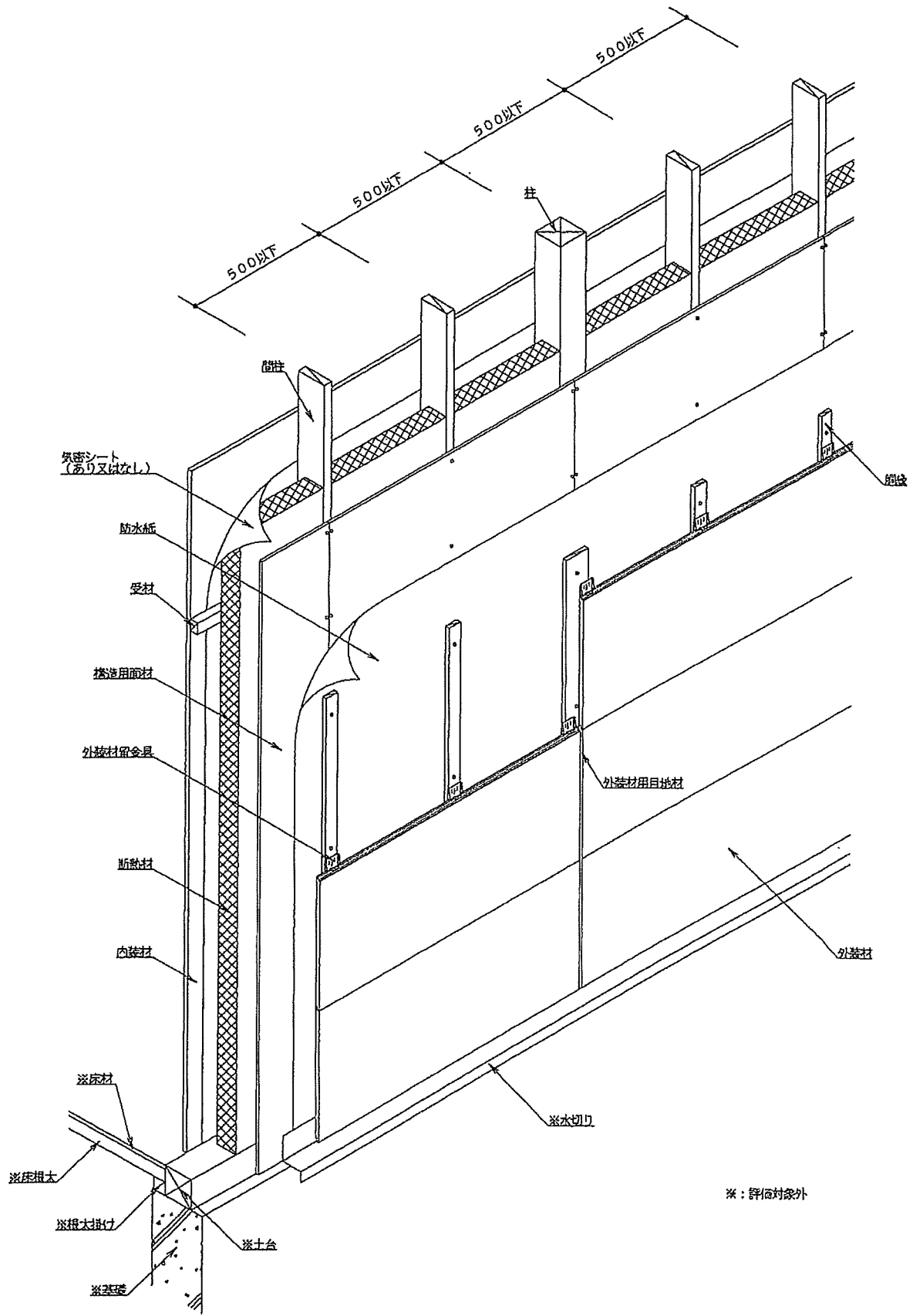
透視図
