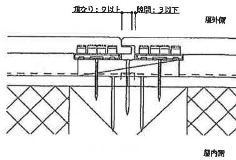
④合いじゃくり目地
