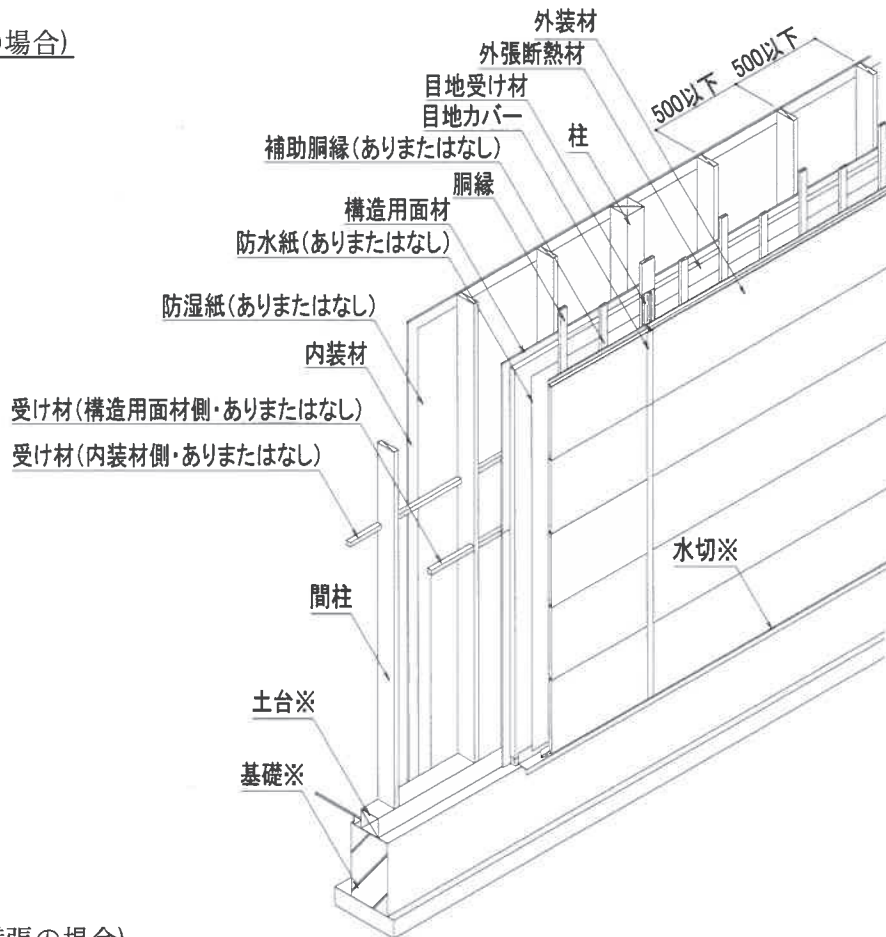
水平断面図 (横張の場合)
