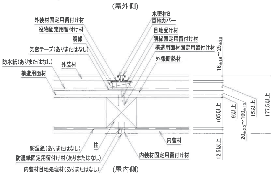
目地部詳細図 (横張の場合・役物：水密材Bあり仕様)
