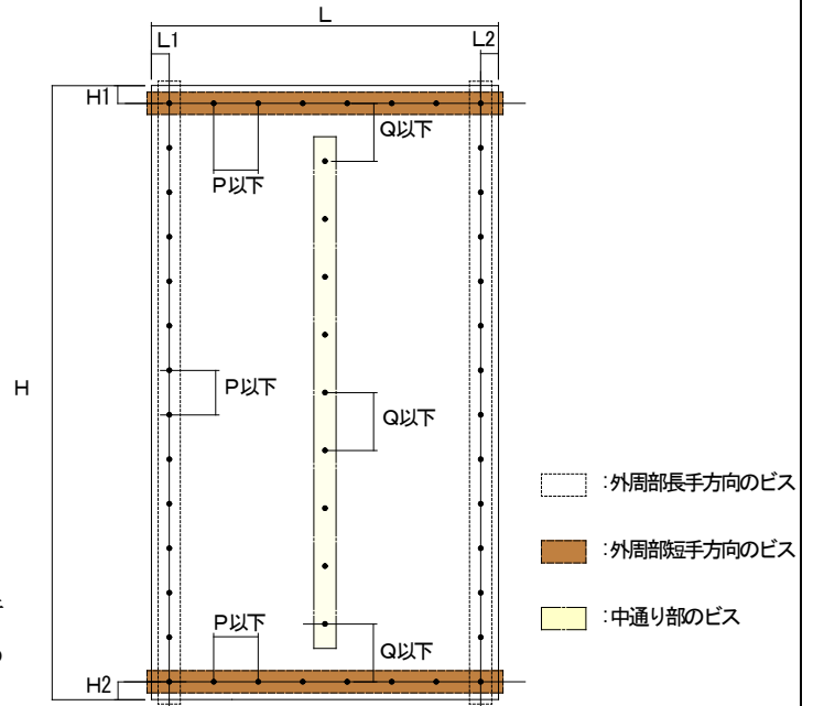
図 ビス留め本
