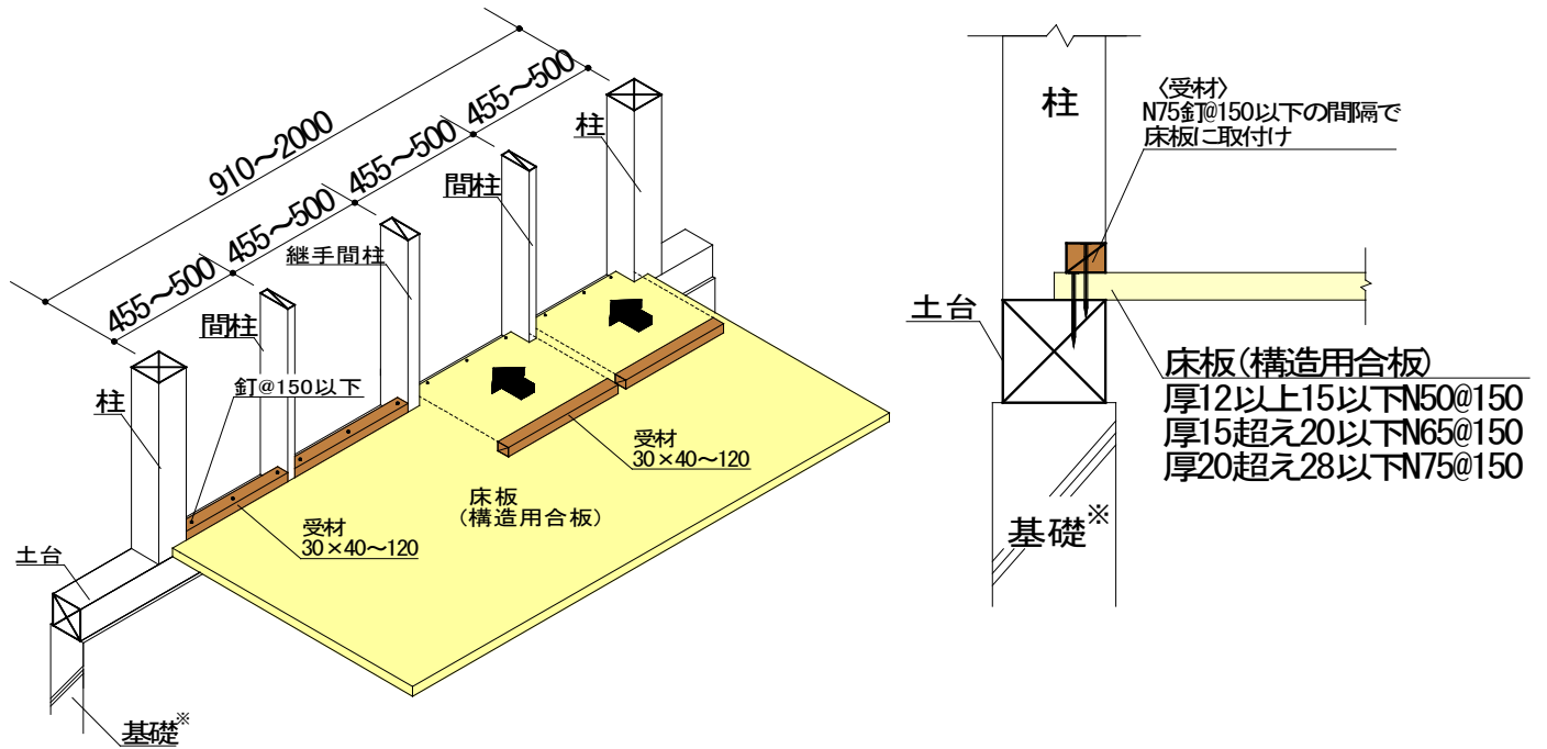
垂直断面図
