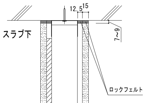
<スラブ下の納まり例>
