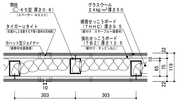
水平断面図
