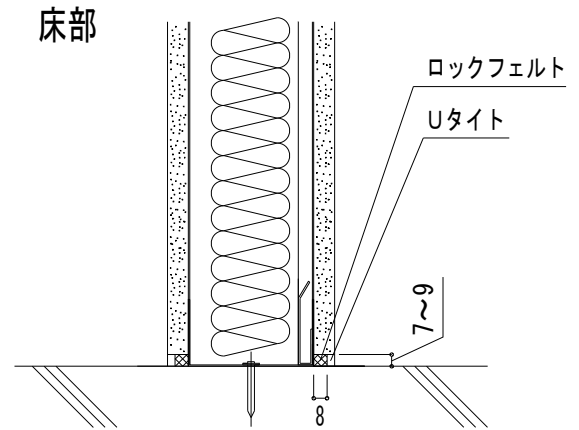
<床部の納まり例>
