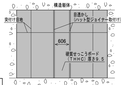
水平断面図
