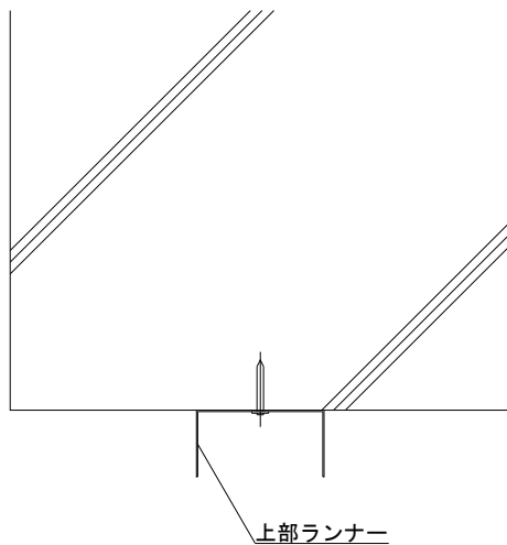
<天井スラブおよびRCへの上部ランナーの取り付け>
