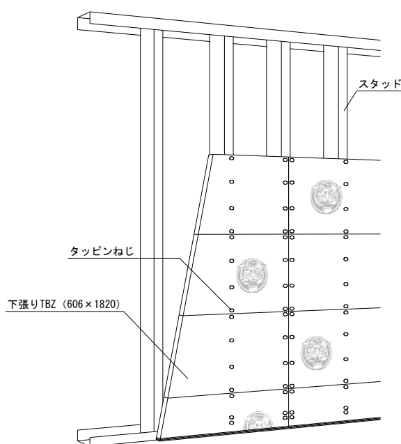
<下張りTBZの張り付け例>
