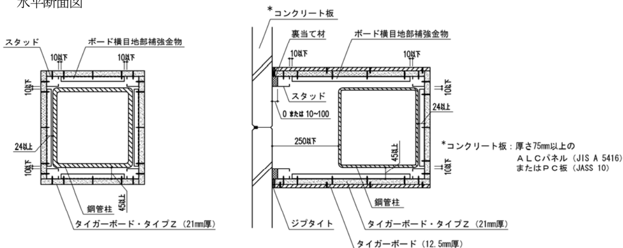
水平断面図
